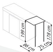
SCHLEPPDACH
